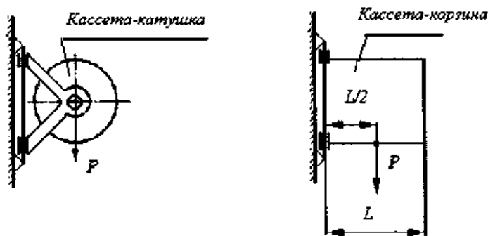
Рисунок 2. Схемы приложения статической нагрузки (P) к поворотной кассете.
