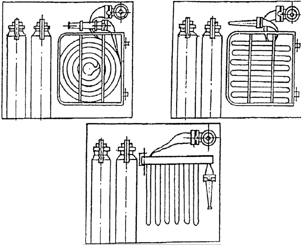
Рисунок 1. Схемы размещения комплектующих изделий в ШП: а - двойная скатка; б - горизонтальная “гармошка”; в - вертикальная “гармошка”
